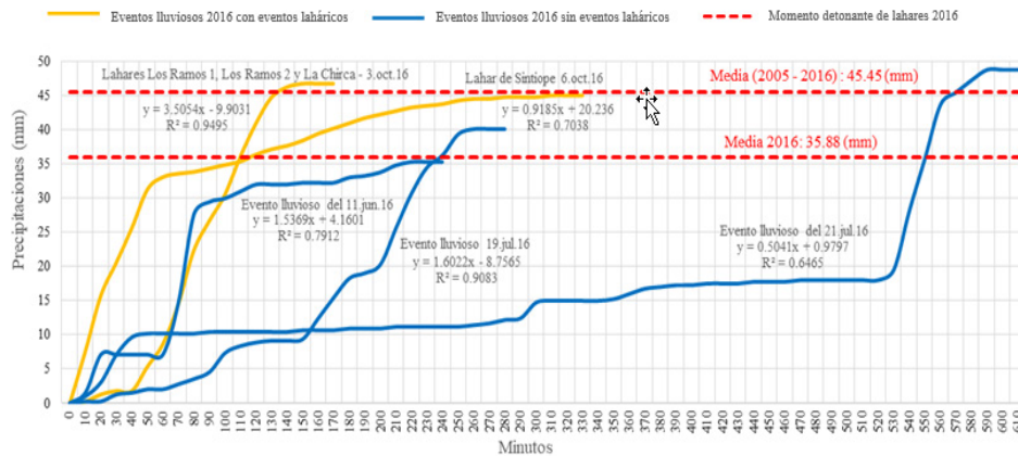
Figura 17. Eventos lluviosos con lahares y eventos lluviosos sin lahares, 2016.
