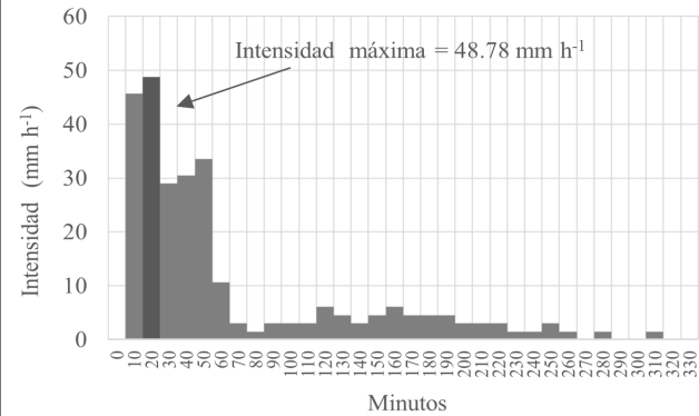
Figura 15. Histograma de intensidad en intervalos de 10 minutos del evento lluvioso del 6.oct.16.
