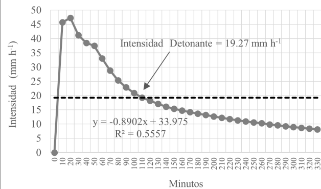
Figura 16. Curva de masa de intensidad del evento lluvioso del 6.oct.16.
