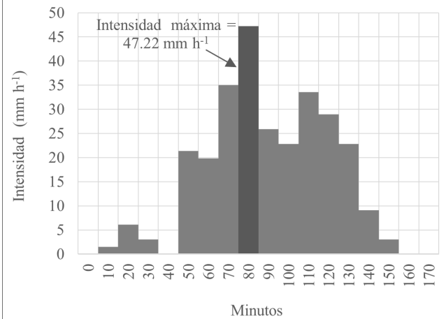
Figura 11. Hietograma de intensidad en intervalos de 10 minutos del evento lluvioso del 3.oct.16.
