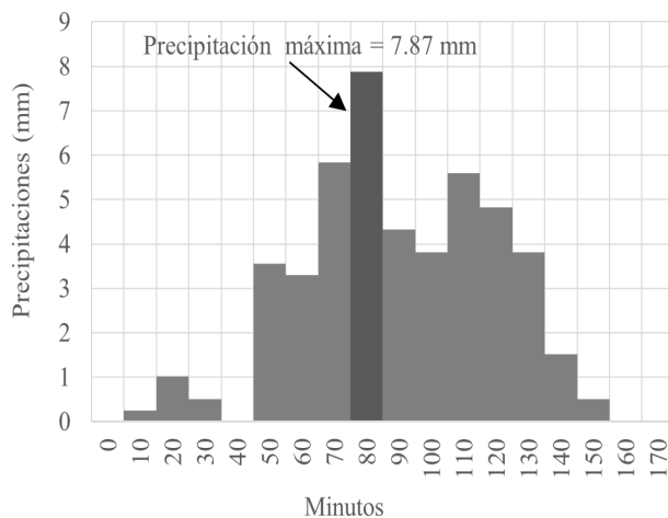
Figura 10. Hietograma de precipitaciones en intervalos de 10 minutos del evento lluvioso del 3.oct.16.
