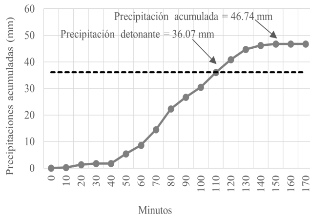
Figura 9. Curva de masa de precipitaciones del evento lluvioso del 3.oct.16.
