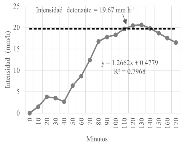
Figura 12. Curva de masa de intensidad del evento lluvioso del 3.oct.16.
