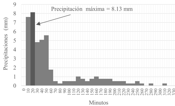
Figura 14. Histograma de precipitaciones en intervalos de 10 minutos del evento lluvioso del 6.oct.16.
