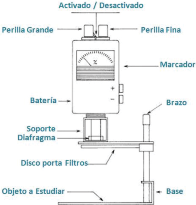
Figura 2. JEULIN Radiómetro, sus partes. Elaboración propia.
