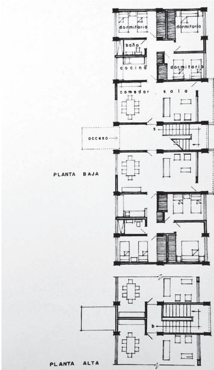
Fig.10. Planta de edificio multifamiliar del Centro Urbano Libertad, San Salvador. Fuente: Memoria 1959-1960 , IVU.
