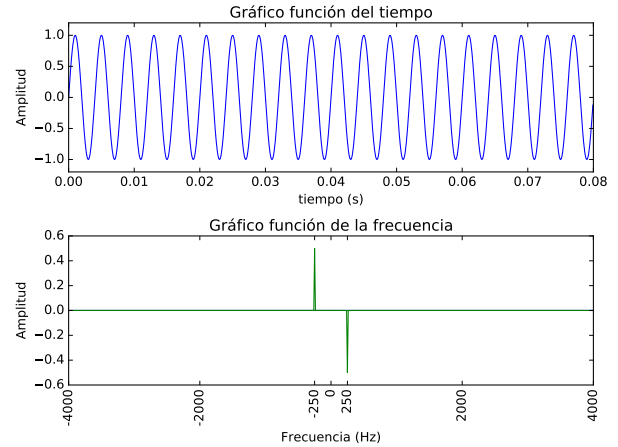
Figura 2: Gráfico de la función A \text{sen}(2\pi f_0 t) y su transformada. A = 1 y f_0 = 250 Hz
